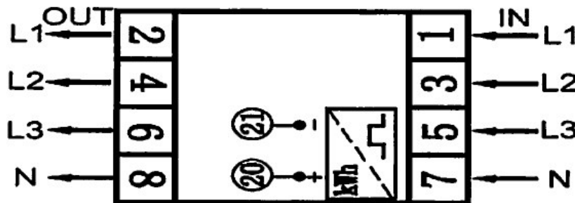
Direktanschluss
